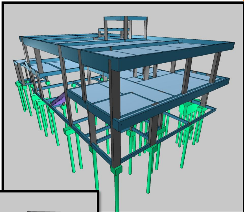
Estrutura de concreto armado para residência com mais de 600m 2 de área construída
