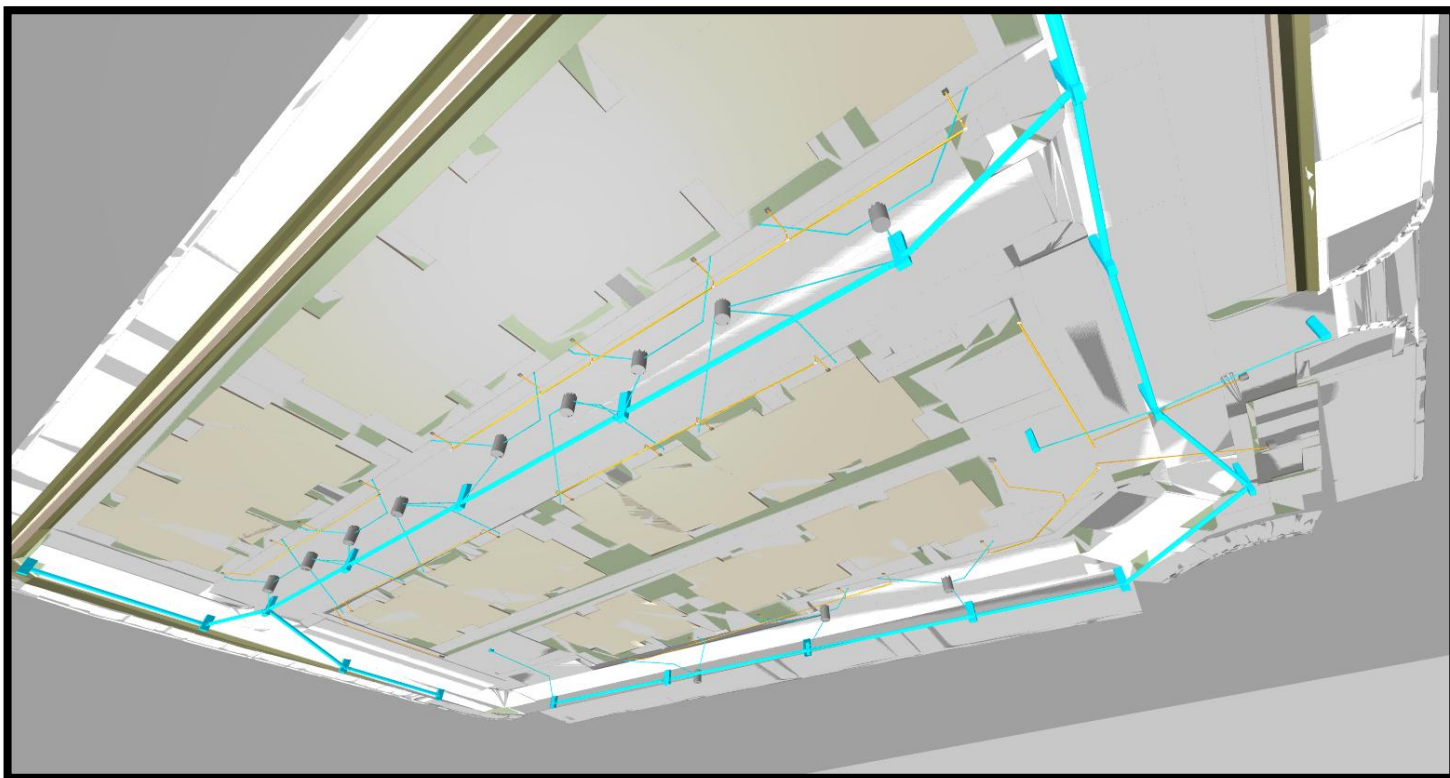
Vista das instalações enterradas de redes de água, esgoto e drenagem de condomínio com 12 torres.
