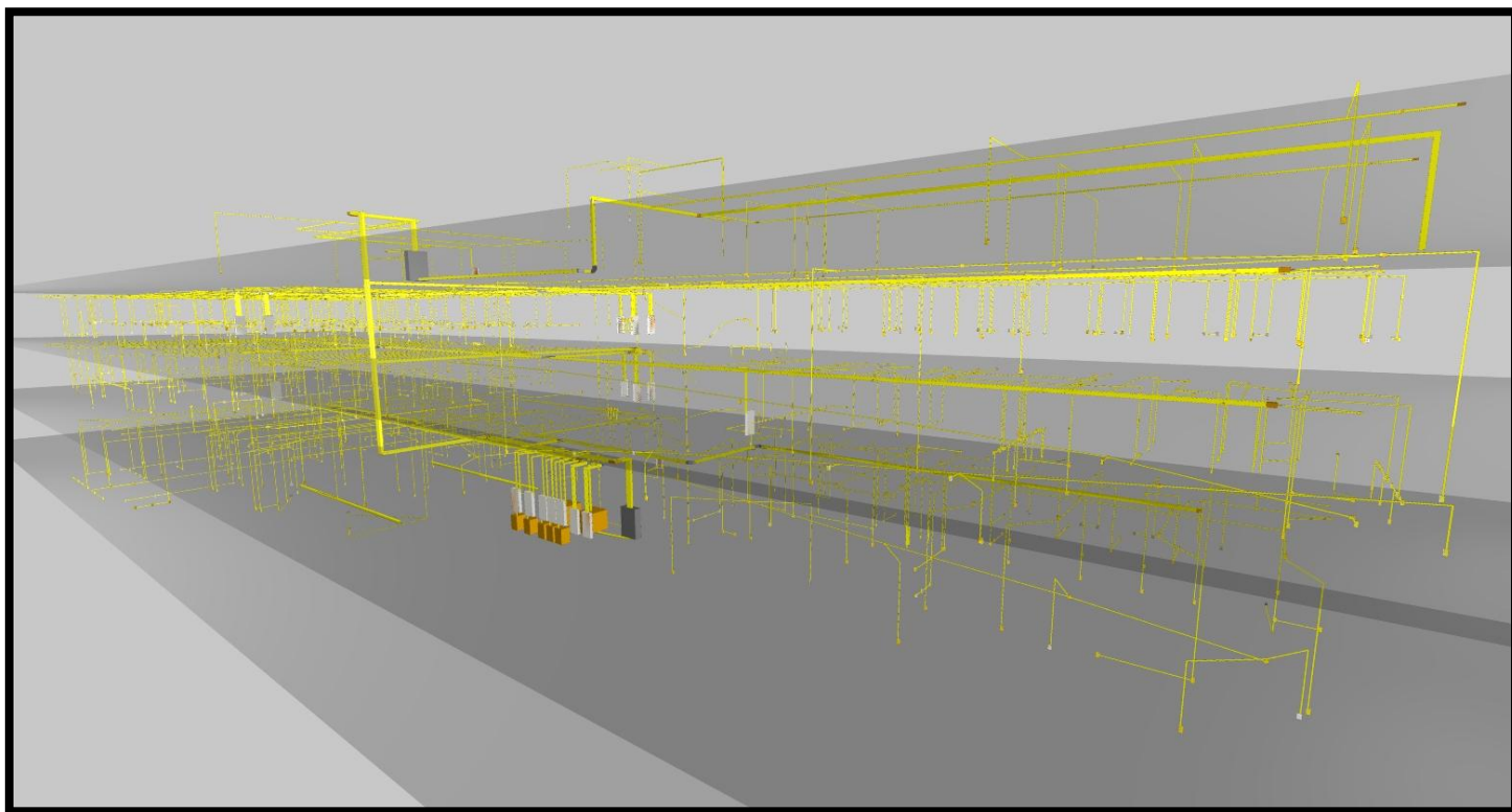
Parte da Modelagem 3D de instalações de Rede Elétrica em Hospital com mais de 10 mil m 2
