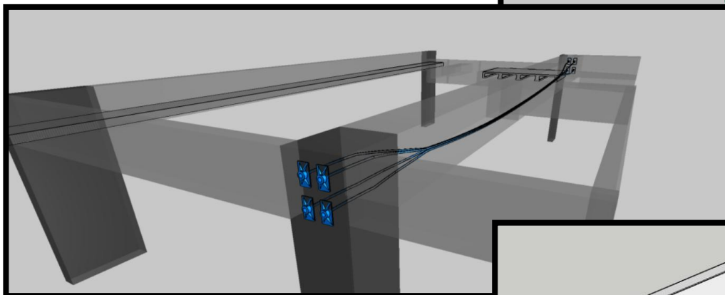
Protensão em concreto armado para vão de 13m em espaço gourmet
