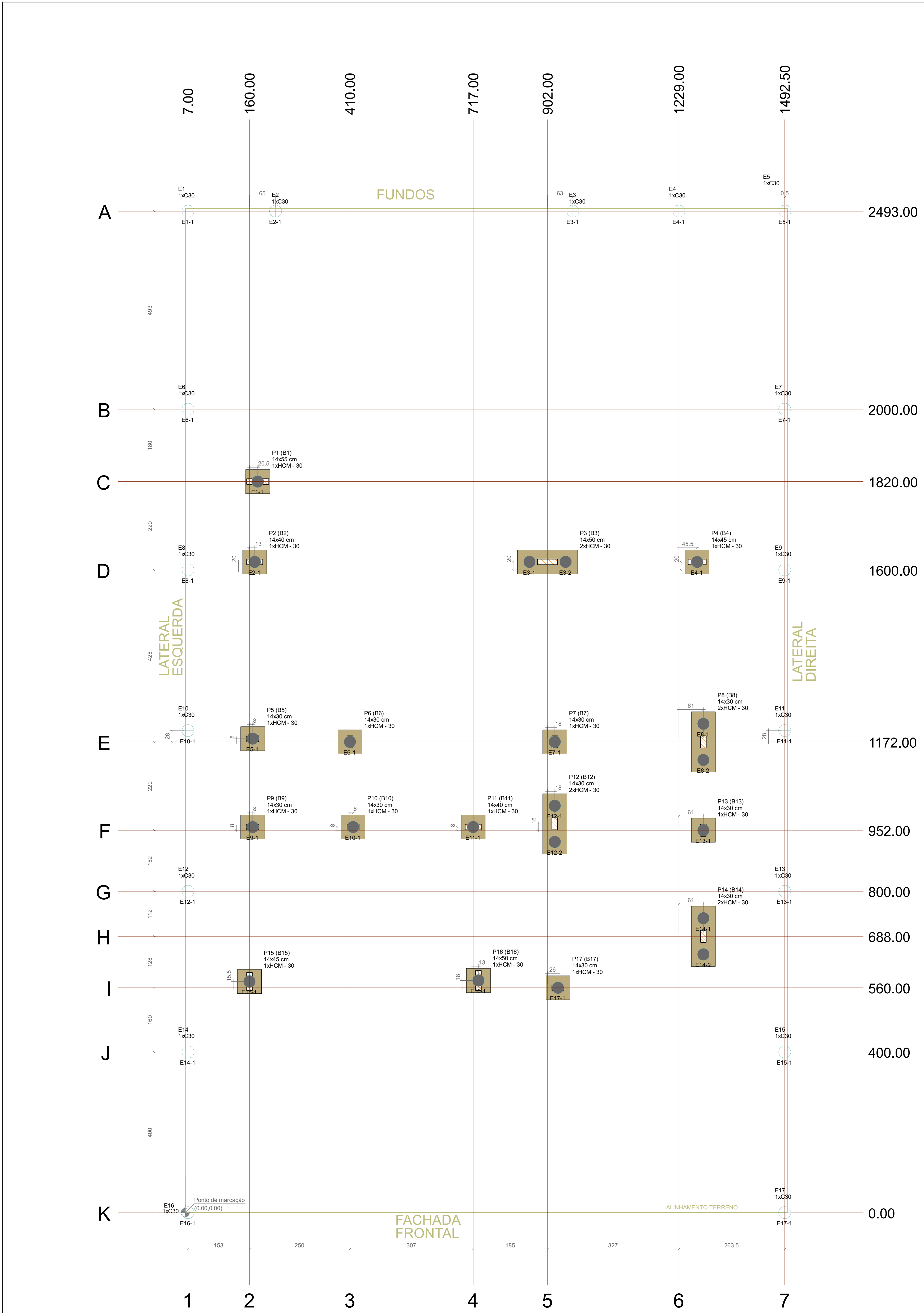
PLANTA DE LOCAÇÃO DAS ESTACAS
